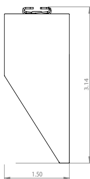
T-Grid 9/16
